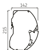
CAPRI cassette
